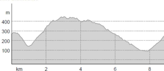
Profilo altimetrico
